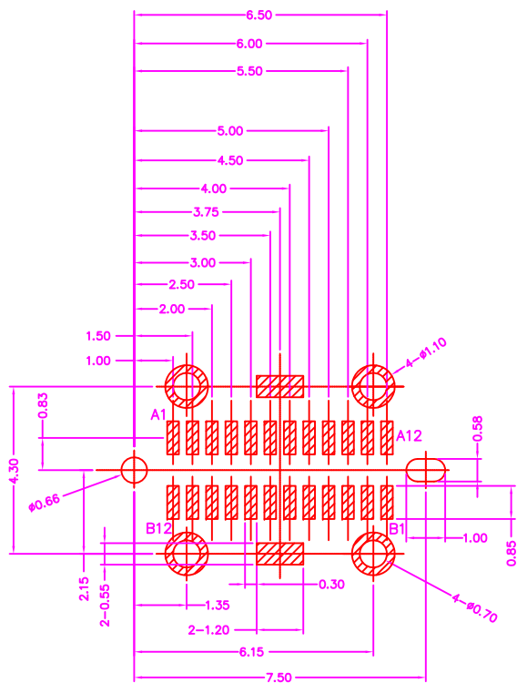
P.C.B. LAYOUT TOP VIEW±0.05 SCALE: 2:1
