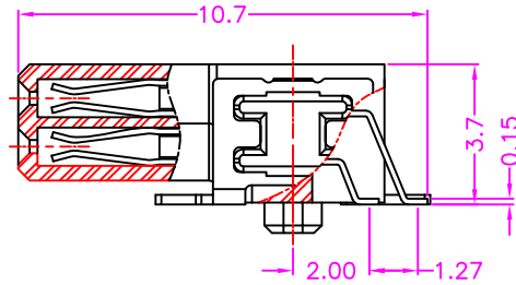
SCALE 2:1
