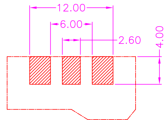
BOTTOM VIEW±0.05
