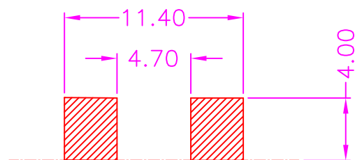
TOP VIEW±0.05
