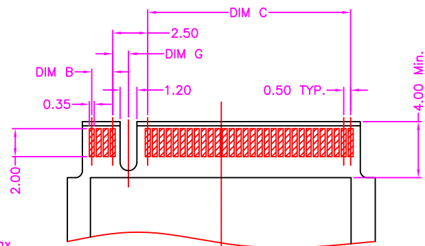
TOP SIDE
