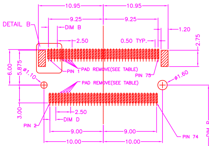
BOTTOM SIDE
