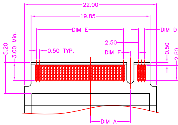
BOTTOM SIDE
